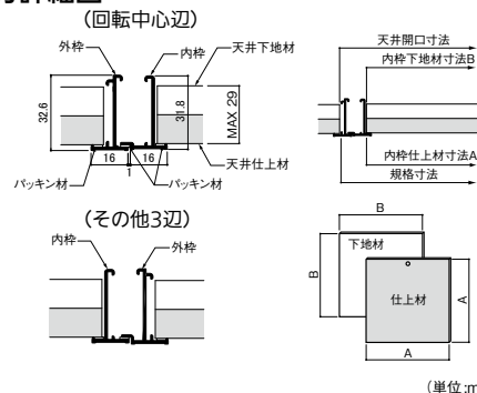
部分詳細図
